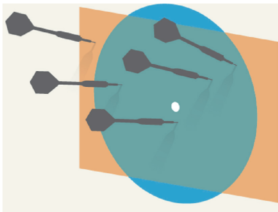
在凸几何中： P(\text{飞镖同时落入圆形和矩形}) \geq P(\text{飞镖落入圆形}) \times P(\text{飞镖落入矩形})
