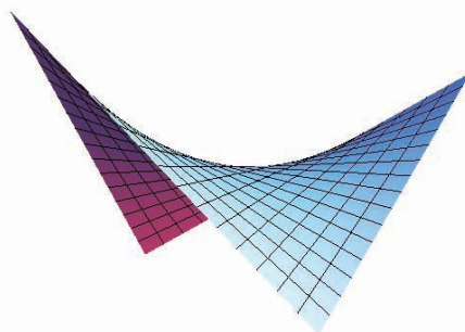
图 2 双曲抛物面
