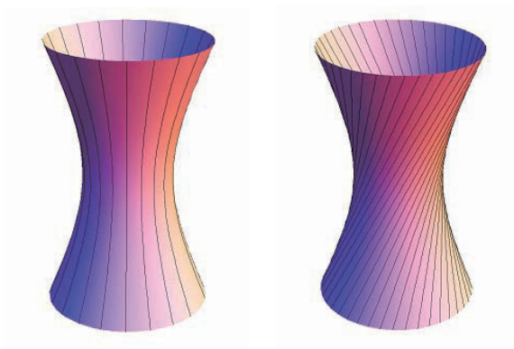
图 4 旋转单叶双曲面: (a) 双曲线绕虚轴旋转 (b) 绕不相垂直的异面直线旋转
